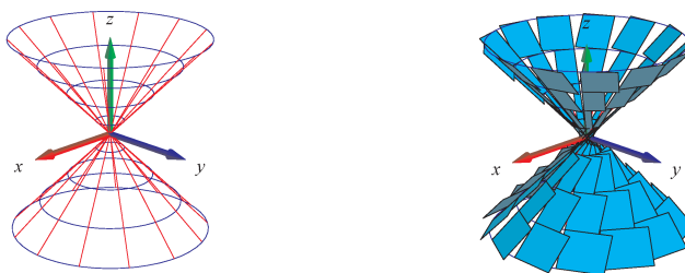
Figur 3.1: Kegle-fladen er givet ved parameterfremstillingen \mathbf{r}(u, v) = (u \cos(v), u \sin(v), u) , u \in [-1, 1] , v \in [-\pi, \pi] . Et system af koordinatkurver på fladen er vist til venstre og de tilsvarende areal-approximerende parallelogrammer er vist til højre. Figureerne er del af output fra Integrator8-kommandoen fladeInt .
