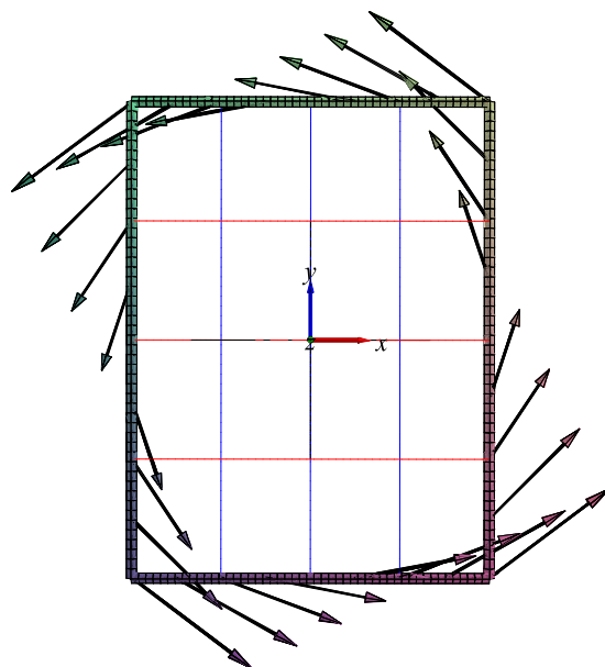
Figur 12.9: Vedrørende eksempel 12.23. Billedets randkurve med antydte vektorfelt \mathbf{V}(x, y) = (-y, x) . Her er valgt et parameterrektangel med a = -1 , b = 1 , c = -1 , og d = 1 . Parameterfremstilling: \mathbf{r}(u, v) = (3u, 4v) . Figuren er output fra kommandoen StokesRandInt .
