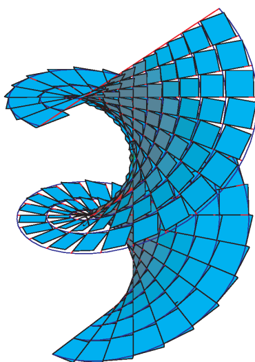
Figur 3.2: Denne vindelflade er givet ved parameterfremstillingen \mathbf{r}(u, v) = (\sinh(u) \cos(v), \sinh(u) \sin(v), v) . Figuren er del af output fra Integrator8-kommandoen fladeInt og viser en approksimation af fladen med parallelogrammer, som faktisk alle er kvadrater af forskellig størrelse. Se opgave 3.8.
