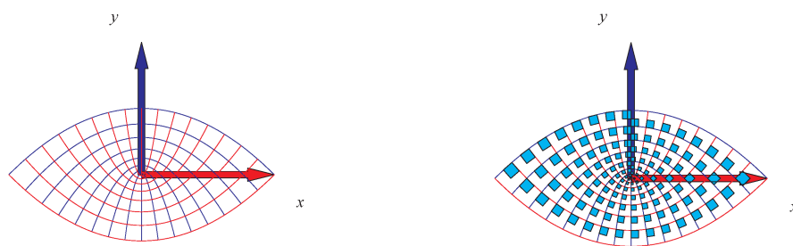
Figur 4.2: Parabelkoordinater. Dette område i planen er givet ved parameterfremstillingen \mathbf{r}(u, v) = (uv, \frac{1}{2}(u^2 - v^2)) , u \in [-1, 1] , v \in [0, 1] . Figuren til højre antyder igen et system af areal-aproksimerende parallelogrammer. Figurerne er del af output fra planIntApprox -kommandoen.
