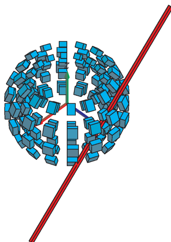
Figur 8.2: En del af en massiv kugle-skål (med tykkelsen 1/4 ) roteres om en akse. Figuren viser placeringer af de approksimerende parallellepipeda i forhold til aksens. Inertimomentet approksimeres af summen af de enkelte deles inertimomenter. Figuren og det eksakte inertimoment af kugleskallen kan beregnes med rumIm -kommandoen.
