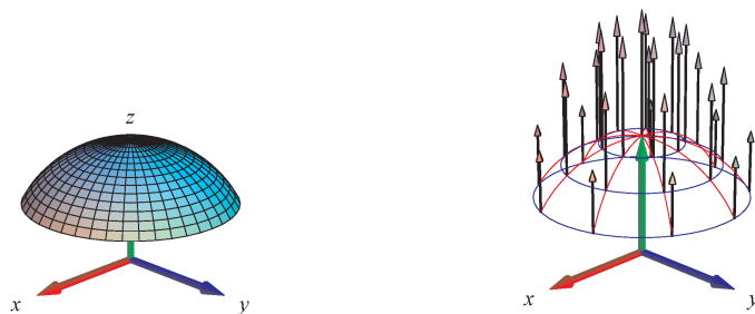
Figur 3.5: Denne kalot af en kugleflade er givet ved parameterfremstillingen \mathbf{r}(u, v) = (\sin(u) \cos(v), \sin(u) \sin(v), \cos(u)) , u \in [0, \frac{\pi}{3}] , v \in [-\pi, \pi] . Vektorfeltet er givet ved \mathbf{V}(x, y, z) = (0, 0, z) . Et system af koordinatkurver på fladen er vist til højre sammen med vektorfeltet evalueret i koordinatkurvernes skæringspunkter. Figureerne er en del af output fra fluxInt -kommandoen anvendt på den givne parameterfremstilling og det givne vektorfelt.
