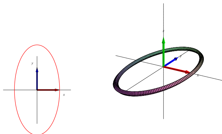
Figur 2.7: En Ellipse med halvakser a = 1 og b = 2 . Se eksempel 2.14.
