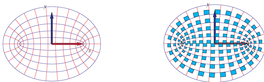
Figur 4.3: Elliptiske koordinater. Dette område er givet ved parameterfremstillingen \mathbf{r}(u, v) = (\cosh(u) \cos(v), \sinh(u) \sin(v)) , u \in [0, 1] , v \in [-\pi, \pi] . Figurerne er del af output fra planIntApprox -kommandoen.
